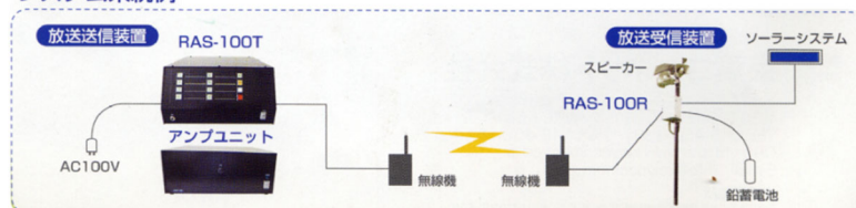
放送受信装置 RAS-100R (ソーラー電源型)
